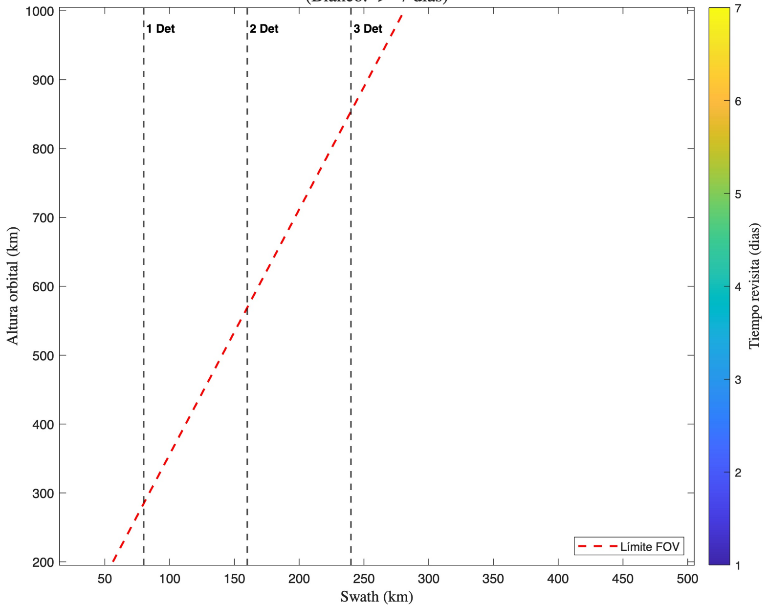
Tiempo Revisita - 1 Satelite(s); 2 Telescopio(s): TMA; Detector 3 (Blanco: > 7 dias)
